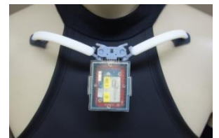
関節角度を計測し、「胸をはる」 「肩をすくめない」を評価する機構
