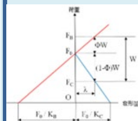
締付け線図
