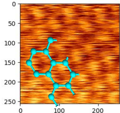
図2 計測したグラファイト(HOPG)表面像
