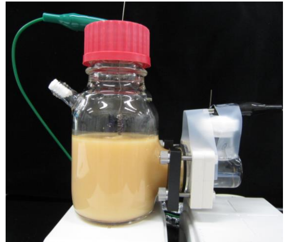
図2 電解中の様子
