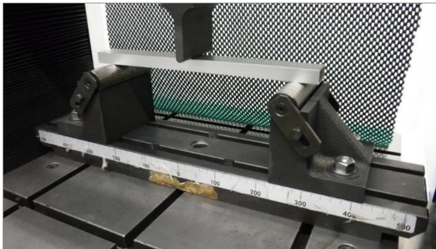
図 1 試験の様子
