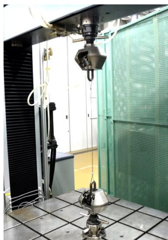
図 1 試験の様子
