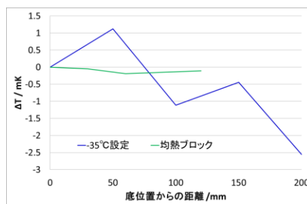
温度分布 (深さ)
