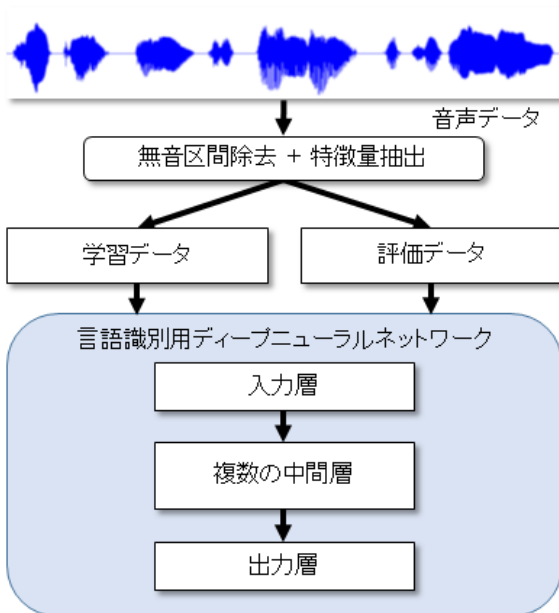
図3. 言語識別処理の流れ
